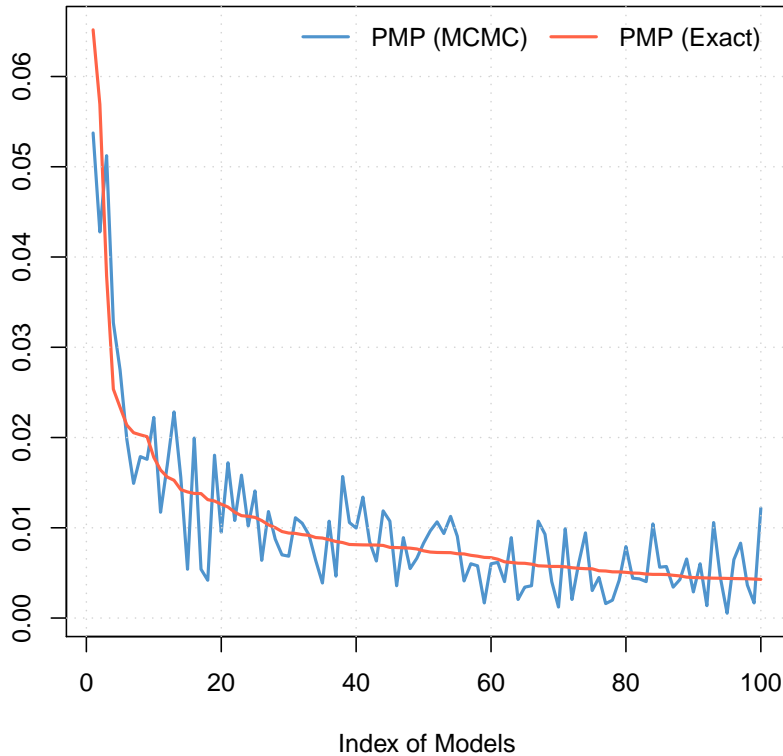
Posterior Model Probabilities (Corr: 0.8920)
