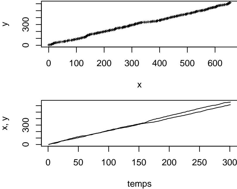
Fig. 1 – Diagramme de dispersion (haut) et chronogrammes (bas) de deux marches aléatoires, x et y , indépendantes.
